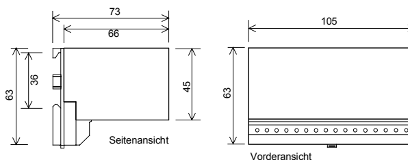
Maßbild 14er Gehäuse in mm
